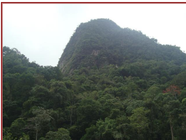
Foto 28. Geoforma conspicua de montañas volcánicas cuya composición litológica corresponde a riolitas y andesitas lavicas. Localidad La Huanca-Cerro La Huanca, Julio 2010.
