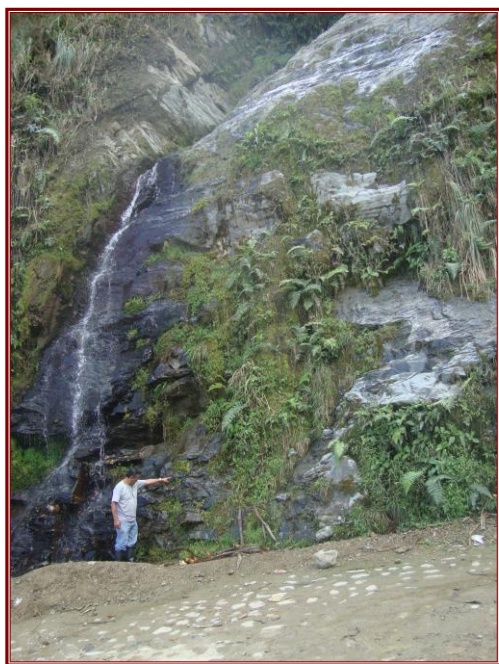
Foto 02. Afloramiento metamórfico de esquistos masivos simulando una tonalidad grisácea por efectos del contacto con el agua. Localizado en el sector San Miguel-Mirador, Julio 2010.
