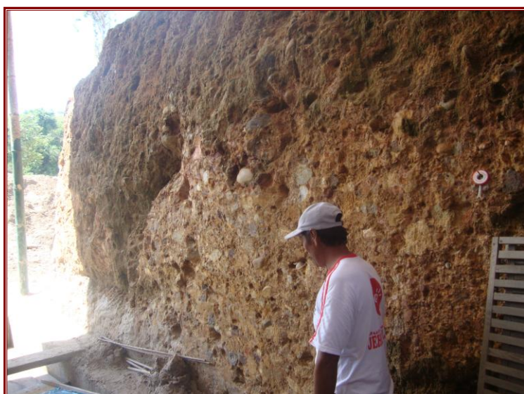
Foto 20. Depósitos aluviales pleistocénicos compuestos por conglomerados de naturaleza polimíctica y heterométrica, dispuestos en potentes bancos. Sector la Esperanza-Aucayacu, Julio 2010.
