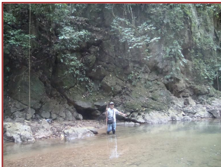
Foto 13. Areniscas masivas de tonalidad gris compactadas altamente fracturadas de la Formación Yahuarango. Sector Catarata-Aucayacu, Julio 2010.
