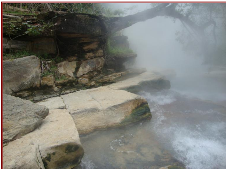
Foto 08. Estratos medianos de areniscas masivas de la Formación Cushabatay, en contacto con las aguas termales. Sector Mayantuyacu-Honoría, Julio 2010.
