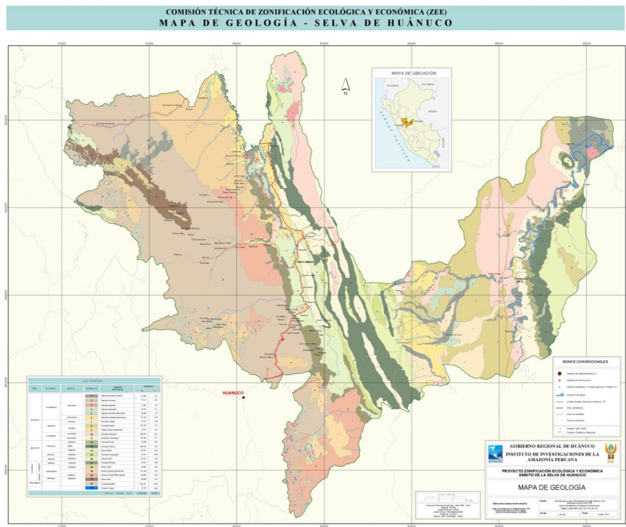
Figura 1. Mapa geológico de la selva de Huánuco.
