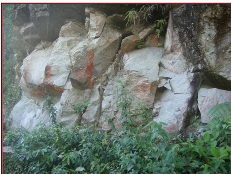
Foto 27. Afloramiento de rocas ígneas intrusivas leucocrata Geoforma con alto contenido de cuarzo, se encuentran conformando las montañas altas. Proximidades de la Localidad de Cholón, Julio 2010.
