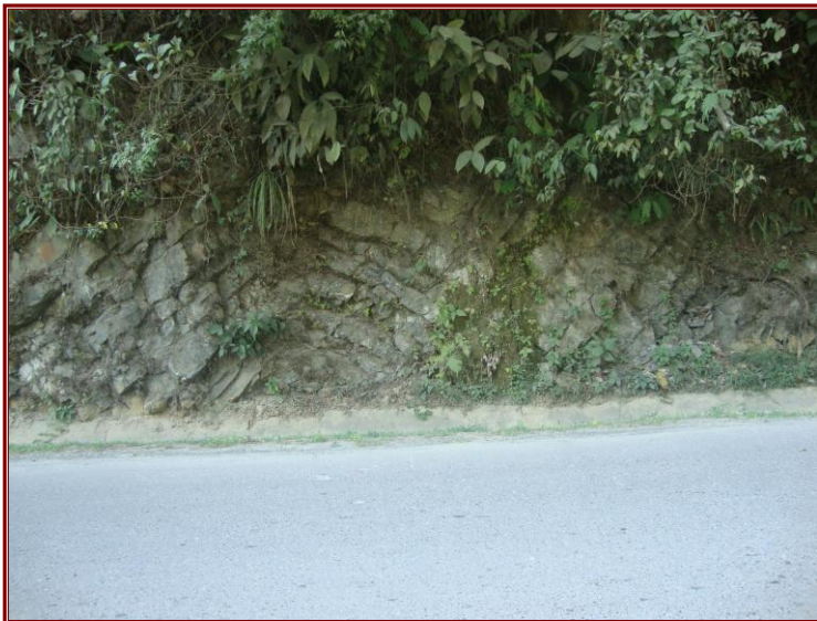
Foto 06. Rocas calcáreas fuertemente plegadas (sinclinal) en estratos delgados, Proximidades de Tingo María, Julio 2010.
