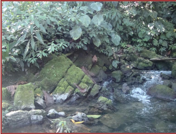
Foto 05. Estratos de calizas en estratos delgados a medianos del Grupo Pucará. Localidad de Consuelo, Julio 2010.
